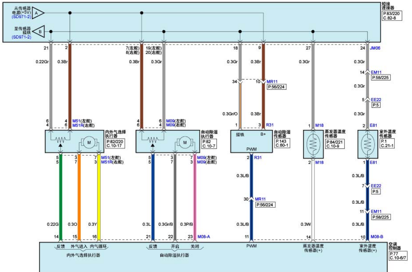
空调控制系统(自动)(3)
